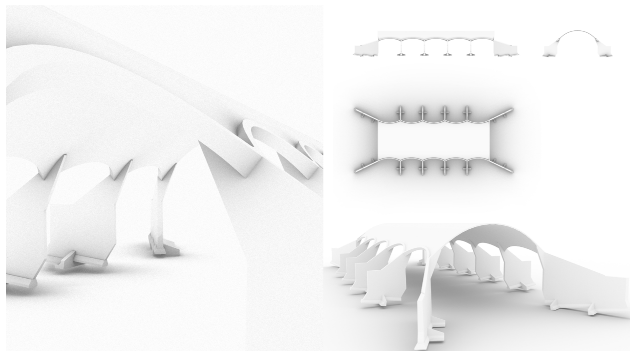
Fig. 7 Mercato dei Fiori, Pescia: structural 3D model of the vault (author: Alice Fantoni).
